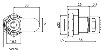
kaba schránkový zámok
