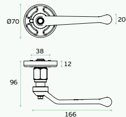
IN.00.390 Puxador de porta com roseta / Door lever handle with rose / Manilla de puerta con roseta.
