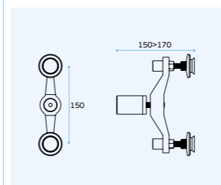
IN.82.005 Suporte para vidro com acessórios / Glass connector with accessories / Soporte para cristal con accesorios.
