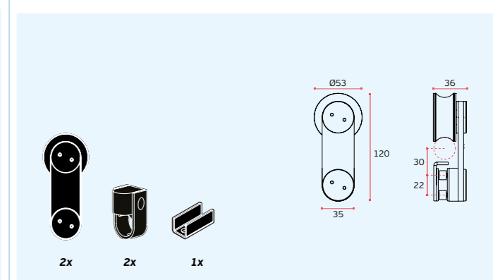
IN.15.601 A2 SYSTEM FOR GLASS
