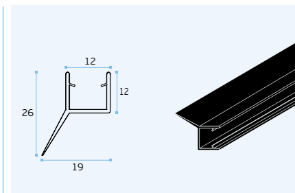
IN.15.998.A (2000mm) Vedante para vidro / PVC seals for glass / Sellos para cristal.
