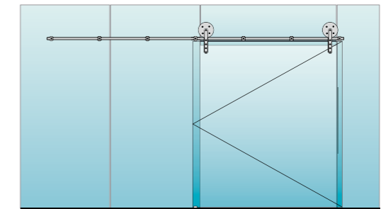
(B) FIXO NO VIDRO / FIXED AT GLASS / FIJO EN Cristal
