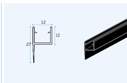
IN.15.998.G (2000mm) Vedante para vidro / PVC seals for glass / Sellos para cristal.
