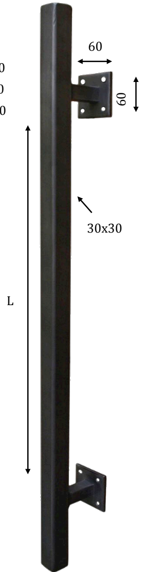
Maniglione Pull handle
