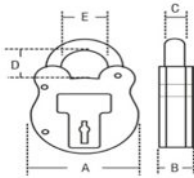
Art.SQ220 A38mm B14,5mm C7mm D11mm E12mm Art.SQ440 A51mm B16,5mm C8mm D18mm E18mm Art.SQ660 A64mm B19,7mm C10mm D21mm E21mm
