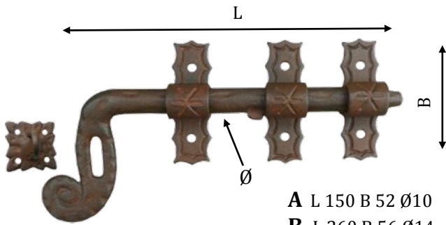
Art. 1021/ Catenaccio portallucchetto Aldrop bolt
